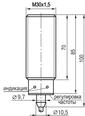
Габаритный чертёж
